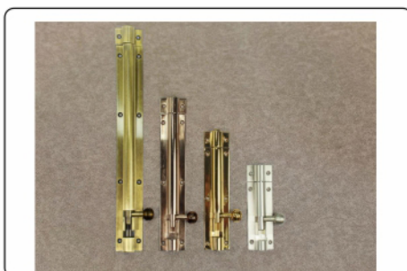
CL-928 (Lotus 12mm Rod) Material : Aluminium +S.S. Finish 4" 6" 8" 12" 18" 24" S.S. 140/- 210/- 280/- 420/- 630/- 840/- AB 152/- 228/- 304/- 456/- 684/- 912/- RG 196/- 294/- 392/- 588/- 882/- 1176/- Gold 196/- 294/- 392/- 588/- 882/- 1176/-
